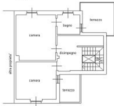
PIANO PRIMO H 2.60 m
